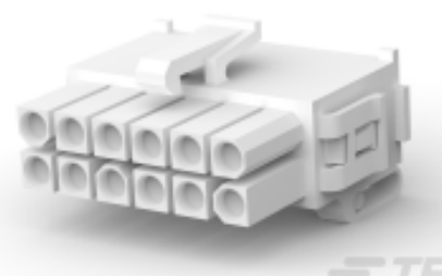
TE Part # 794198-1 12P MINI UMNL2 PLUG HSG DBLROW
