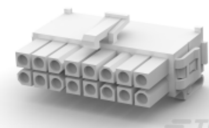
TE Part # 794206-1 16P MINI UMNL2 PLUG HSG UL94V0
